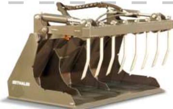
Sperrgutschaufel mit Aufsatz Bucket (open sides) + grabber
