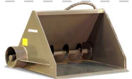
Futterdosierschaufel Feed dosing bucket
